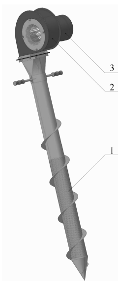
Рис.1 – Общий вид аэратора.
